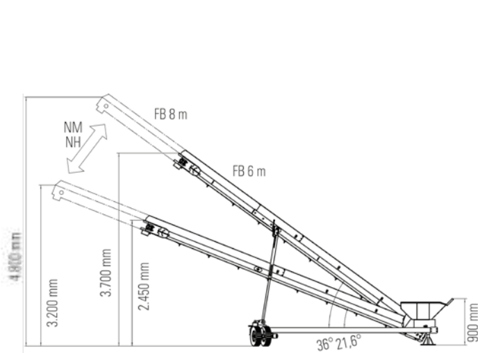
Förderband 6/8 m FSX Seitenansicht
