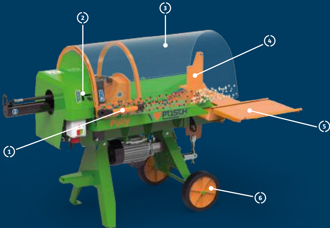
Polly mit serienmäßigem 4-fach-Spaltmesser
