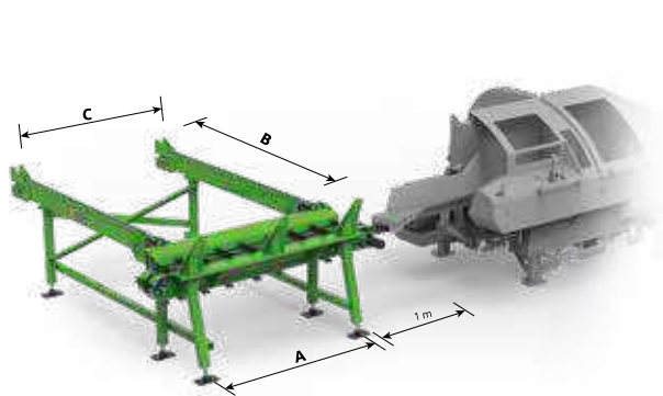
Stammfördersystem
