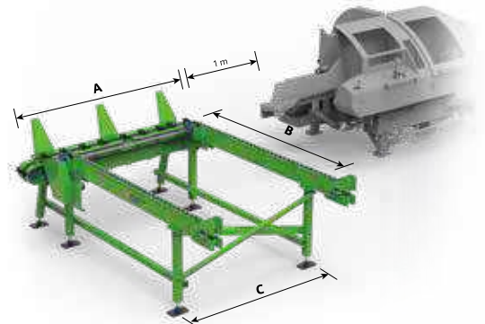
Stammfördersystem mit bedienerseitigem Anbau des Querförderers (Option B)
