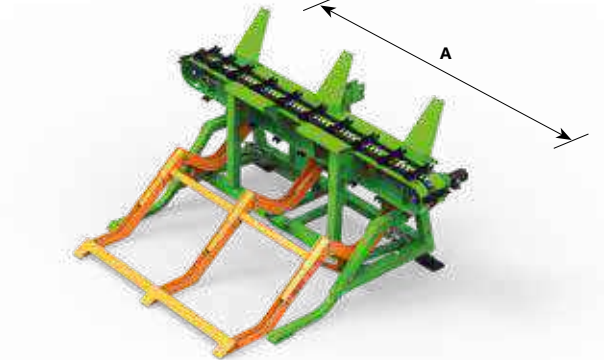
Kettenlängsförderer mit Stammheber (Artikel-Nr. F0002227EDH)
