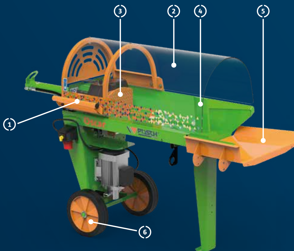
Oscar (E3-400-R) mit serienmäßigem 2-fach-Spaltmesser
