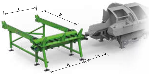
Stammfördersystem
