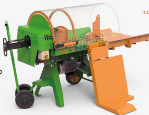
Polly E5,5-R mit serienmäßigem 4-fach Spaltmesser und optionaler Hebevorrichtung
